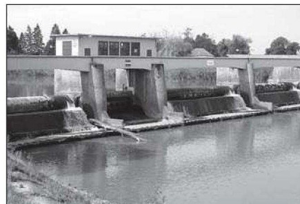
A nicki duzzasztómű
